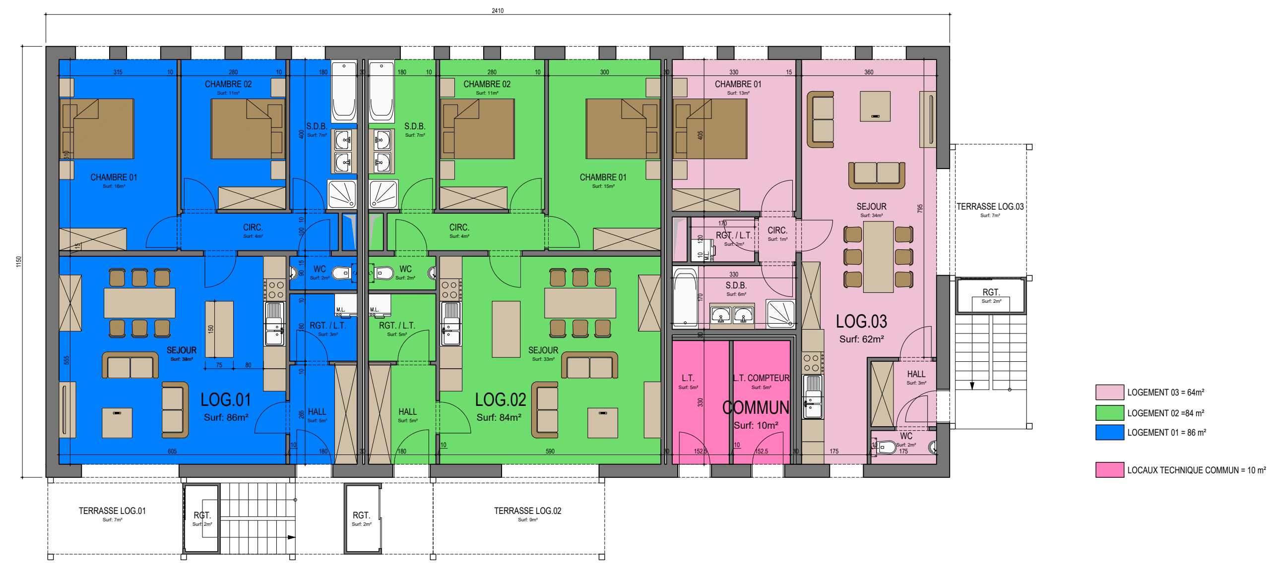
PLAN REZ-DE-CHAUSSEE
